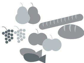
ნოყიერი საკვები
