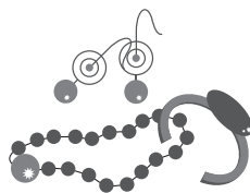
სამკაულები
