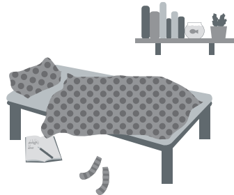
საკუთარი საძინებელი
