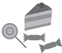
ტკბილეულობა
