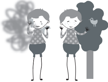
სუფთა გარემო
