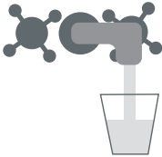
სუფთა წყალი
