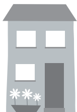
კომფორტული საცხოვრებელი
