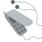
მობილური ტელეფონი
